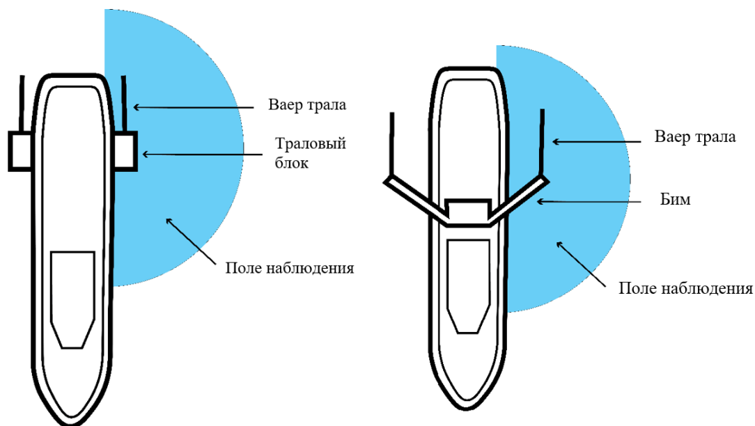
Рисунок 1: Поля наблюдения радиусом 25 м. для подсчета численности морских птиц на судах с традиционным кормовым тралом (слева) и бим-тралом непрерывного лова (справа). Положение указанных объектов может быть разным, в зависимости от судна. Масштаб на рисунках не соблюден.
